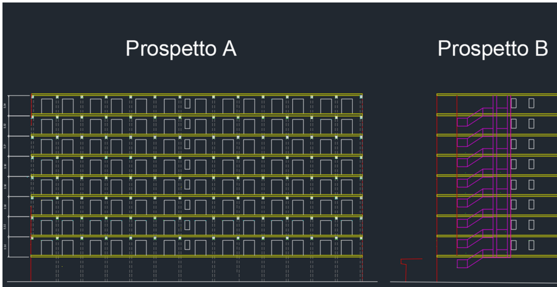
PROSPETTO COMPLETO DELLA FACCIATA
